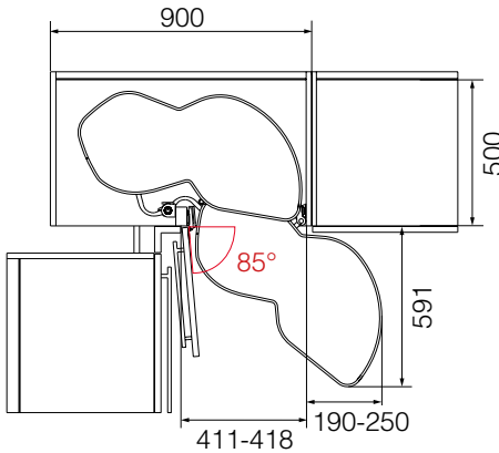
DESTRO ANTA 450MM
