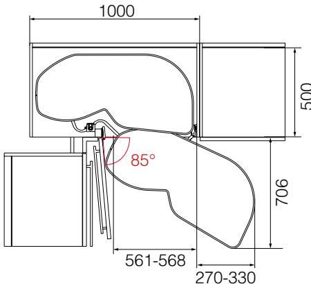
DESTRO ANTA 600MM
