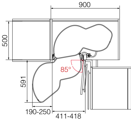
SINISTRO ANTA 450MM
